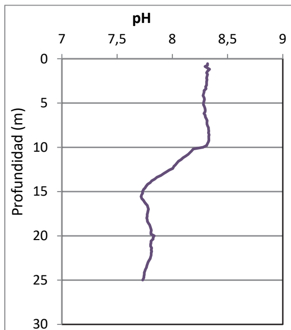
Figura 2. Perfil vertical de la temperatura y pH.
