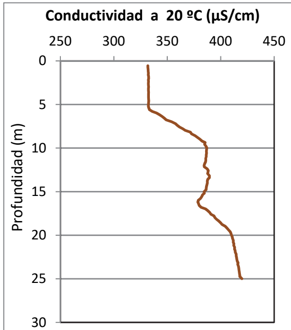
Figura 4. Perfil vertical de la conductividad.
